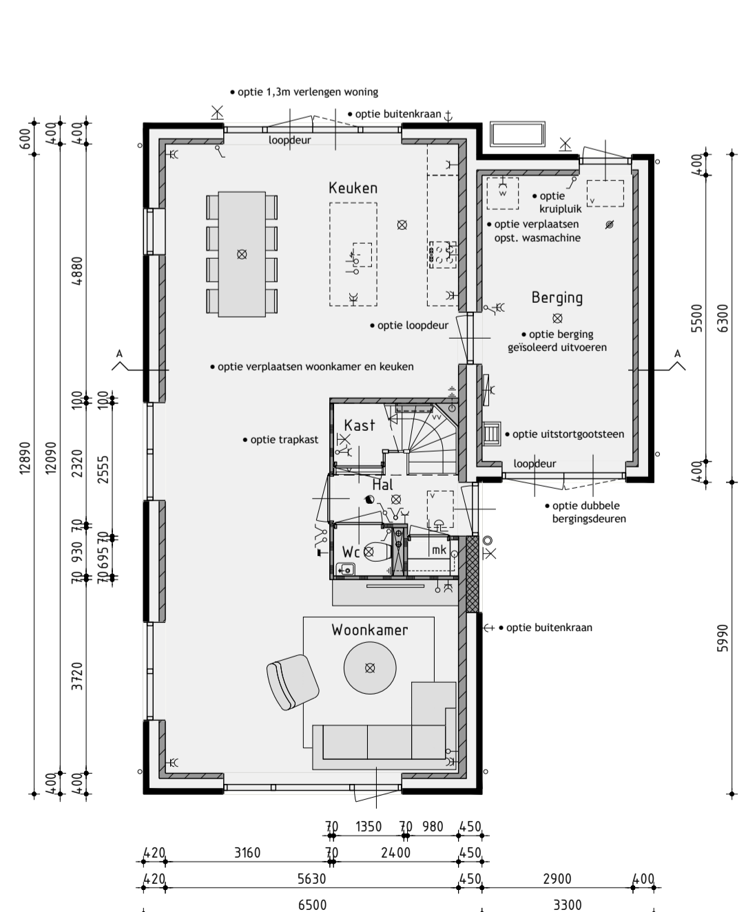
Begane grond v.z.v. vloerverwarming exclusief berging
