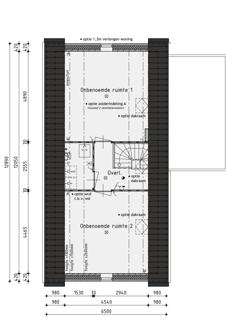
2de Verdieping v.z.v. vloerverwarming de onbenoemde ruimten voldoen niet aan de eisen voor het verblijven van personen op het gebied van o.a. daglicht, ventilatie, hoogte boven de trap, plafondhoogte en boilerinhoud van de warmtepomp.
