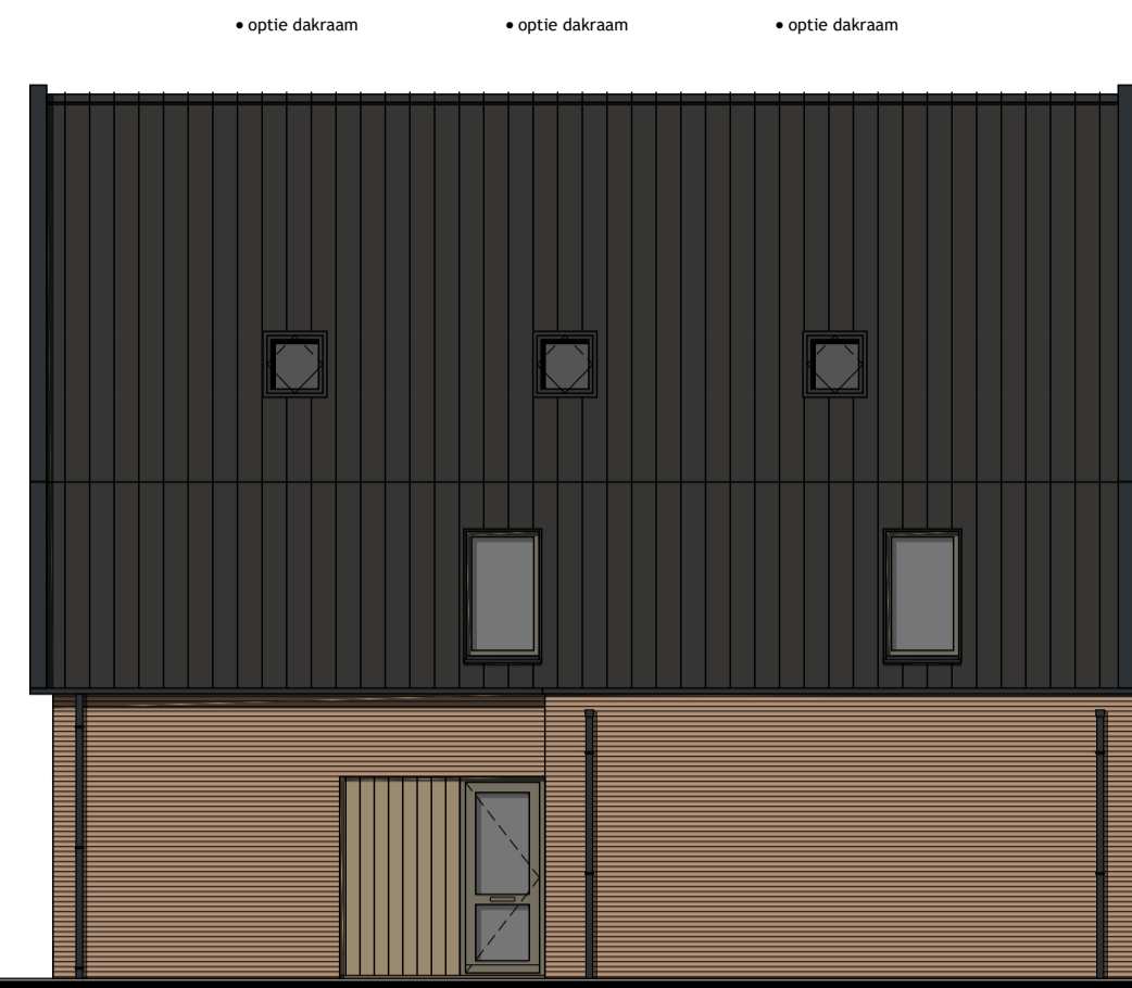
Rechter zijgevel
